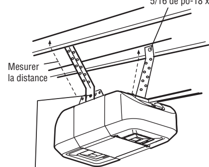
Boulon hexagonal de 5/16 de po-18 x 7/8 de po, Rondelle frein de 5/16 de po, Écrou de 5/16 de po-18
