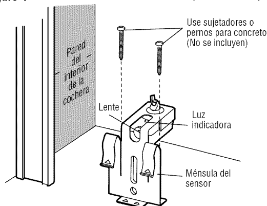
Figura 4 INSTALACIÓN EN EL PISO (LADO DERECHO)
