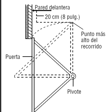
Puerta de una sola pieza sin carril: tornillería del pivote
