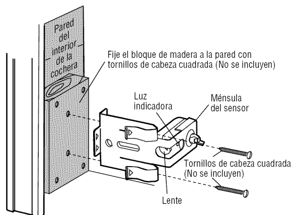
Figura 3 INSTALACIÓN EN LA PARED (LADO DERECHO)
