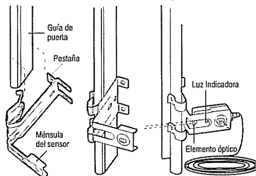
Figura 1 MONTAJE DE GUÍA DE PUERTA (LADO DERECHO)
