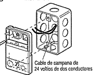
Figura 2 INSTALACIÓN PRECABLEADA
