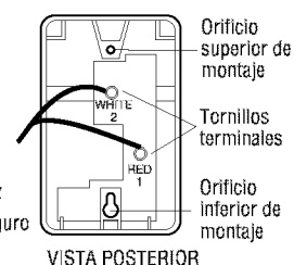
Figura 2 INSTALACIÓN PRE-CABLEADA
