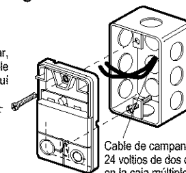
Figura 2 INSTALACIÓN PRE-CABLEADA
