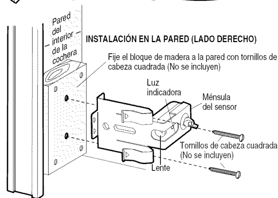
Figura 3 INSTALACIÓN EN LA PARED (LADO DERECHO)
