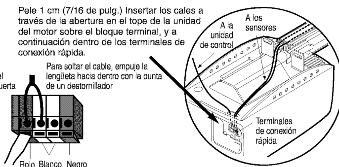
Figura 3 Cableado al bloque de terminales del motor
