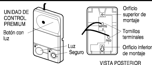
Figura 1 QUITAR Y VOLVER A PONER LA TAPA Para volver a ponerla, primero inserte las lengüetas superiores
