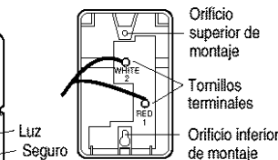
Figura 2 INSTALACIÓN PRECABLEADA
