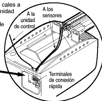
Figura 3 Cableado al bloque de terminales del motor
