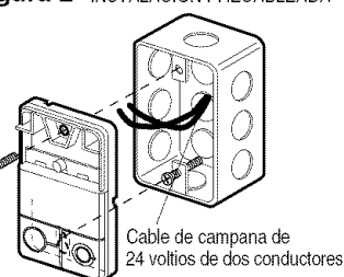
Figura 2 INSTALACIÓN PRECABLEADA
